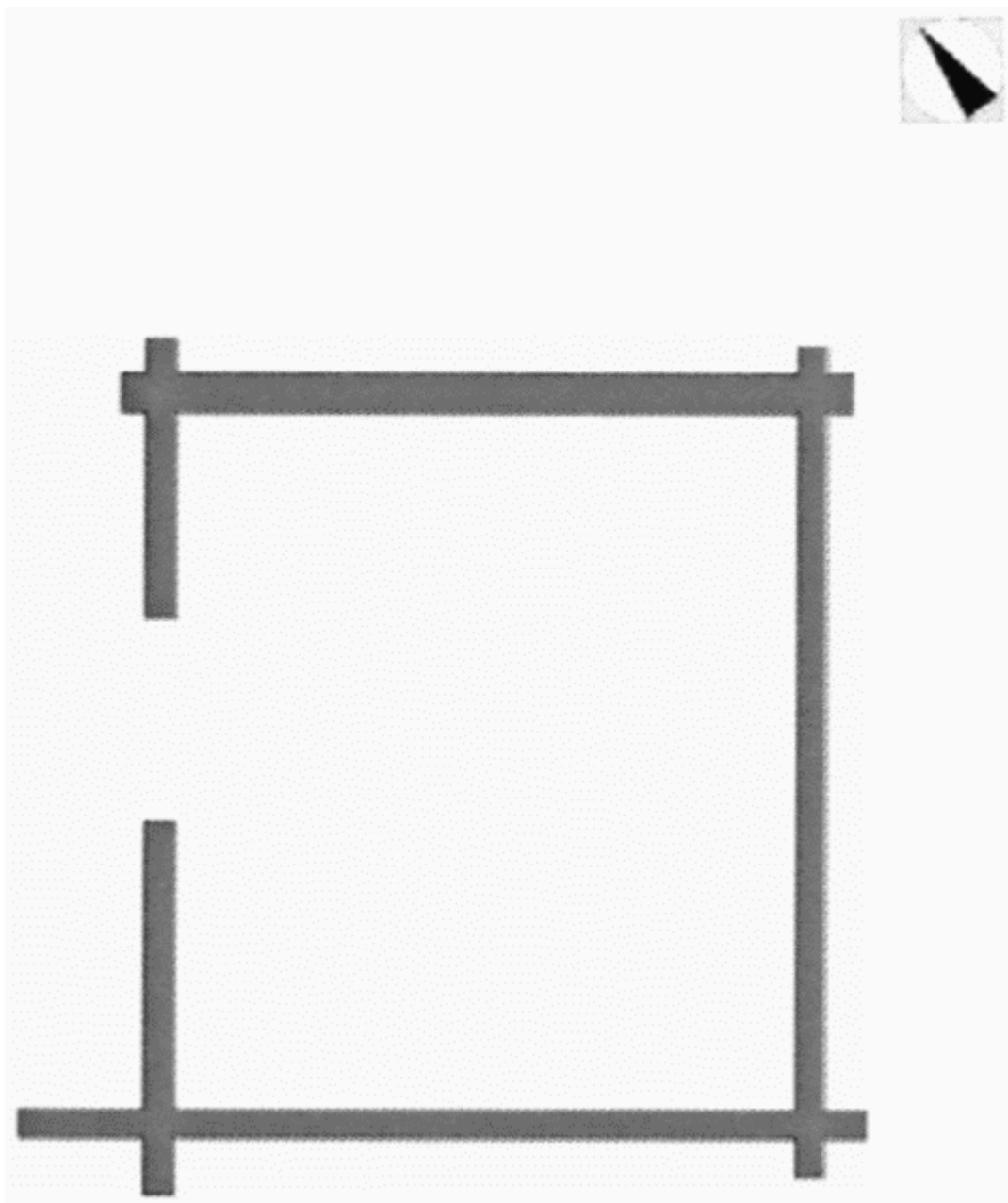
ПЛАН ЛЕДНИКА
