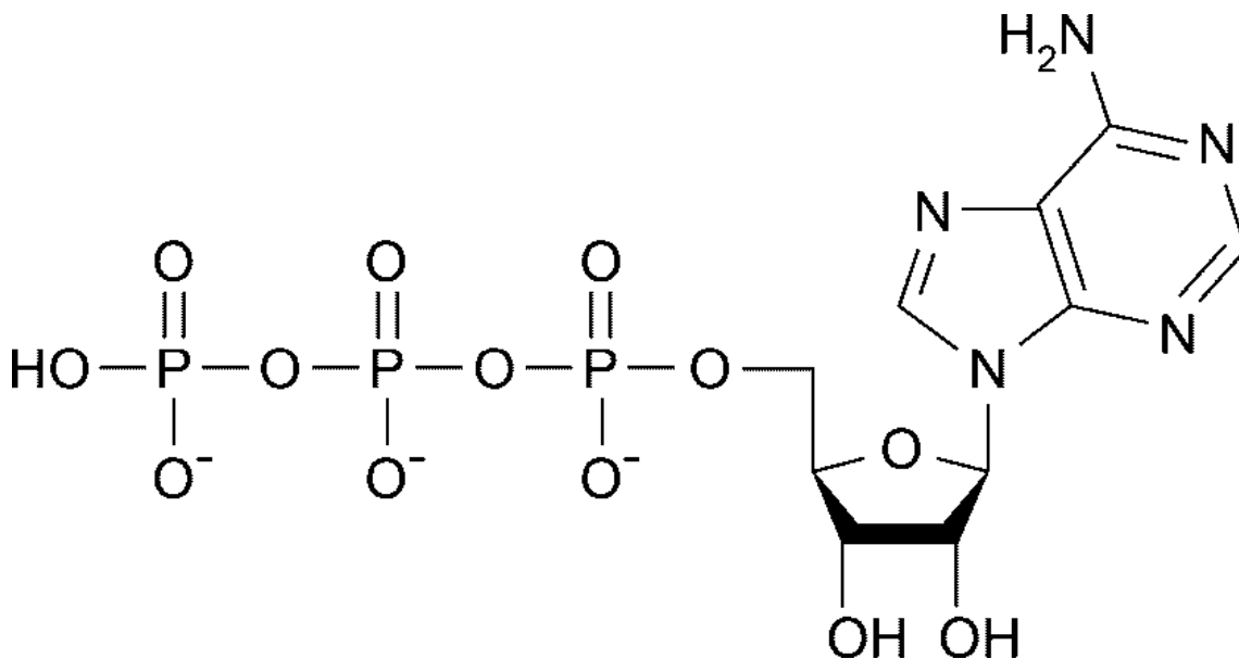
Рисунок А.1 – Молекулярное строение АТФ
